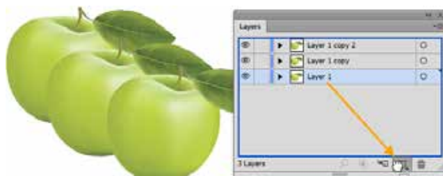
Duplicate Layer
