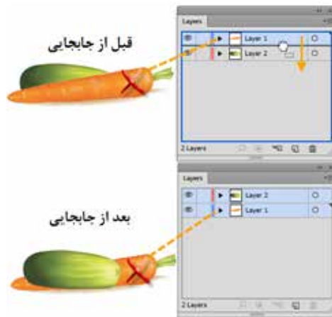
شکل ۵-۱۰ جابجایی لایه‌ها
